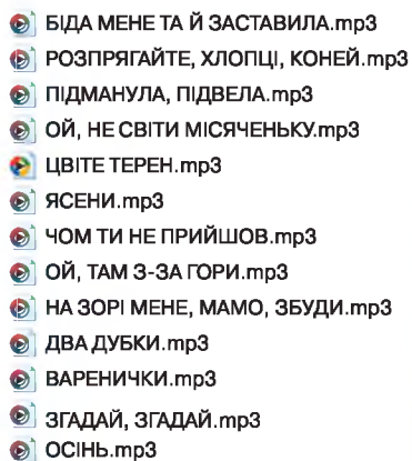
Рис. 2.20. Список файлів
