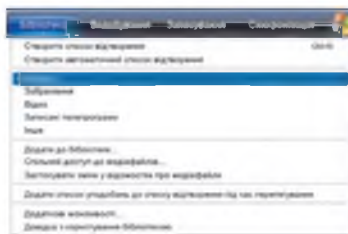
Рис. 3.27. Меню Бібліотека
