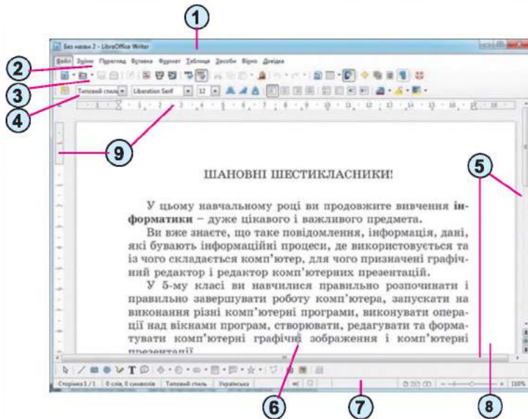
Рис. 4.2. Вікно Writer
